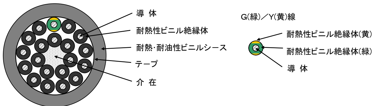
断面図（20心）
