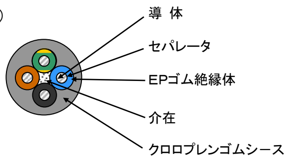
断面図（4心）
